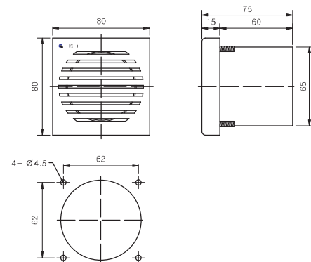
결선도 (Connection Diagram)
