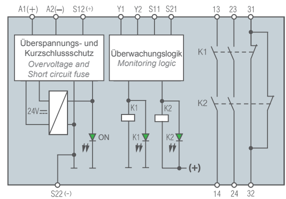
Blockschaltbild Block diagram
