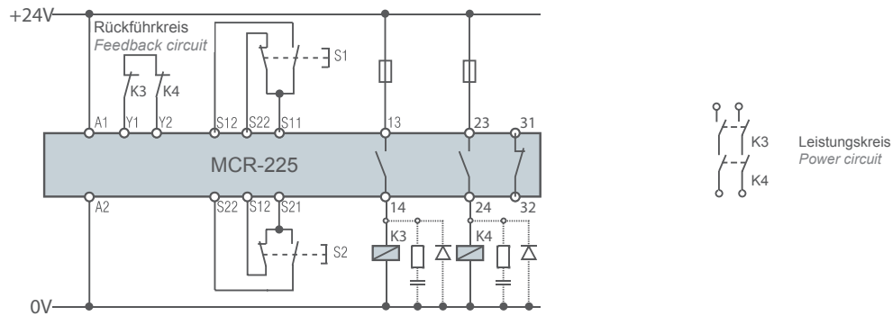
Anschlußübersicht mit Kontaktvervielfältigung Connection diagram with contact multiplication
