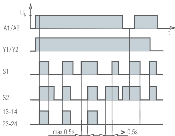
Funktionsdiagramm Functional diagram
