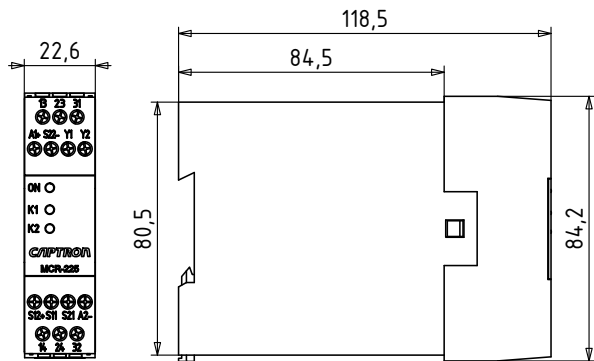
Maßzeichnung Drawing
